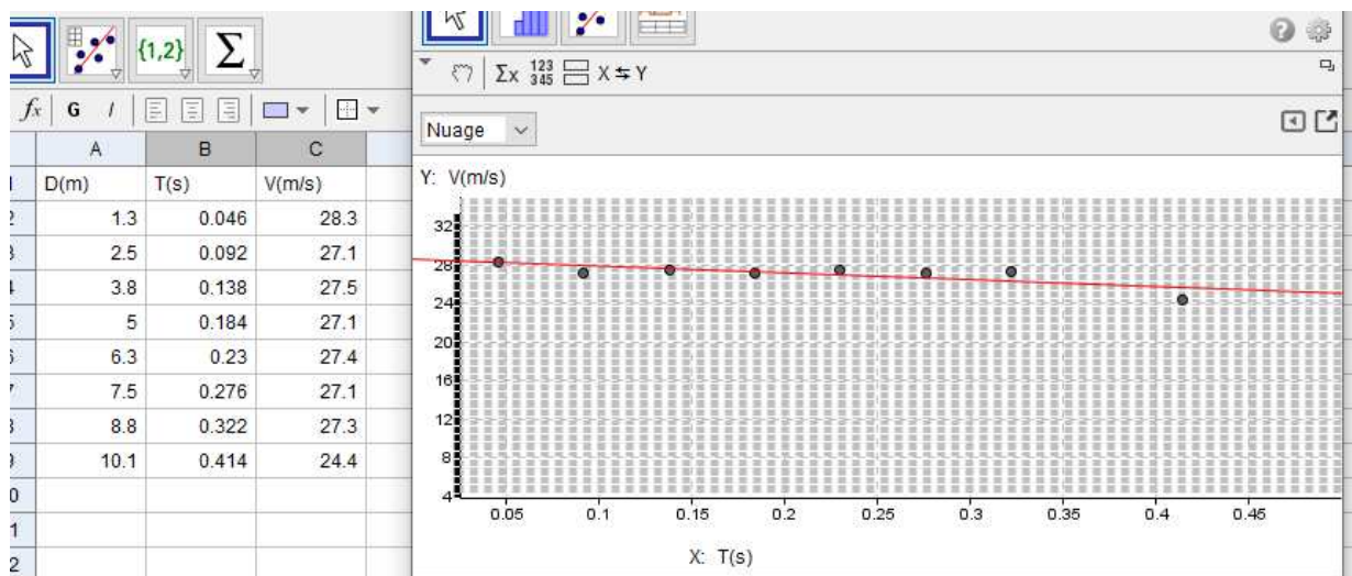
Image 1: mouvement uniforme
